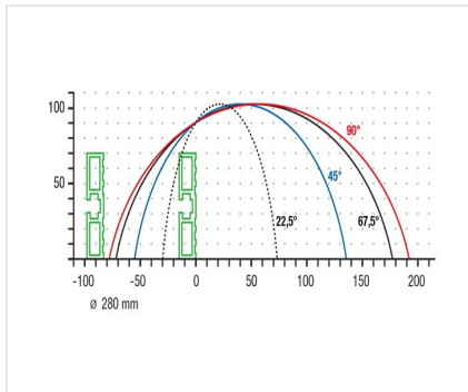
台式锯床TS 161/21
