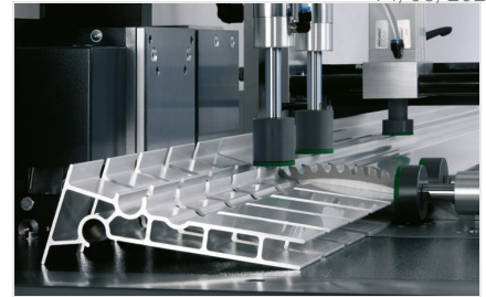
自动锯切机SA 142/38
