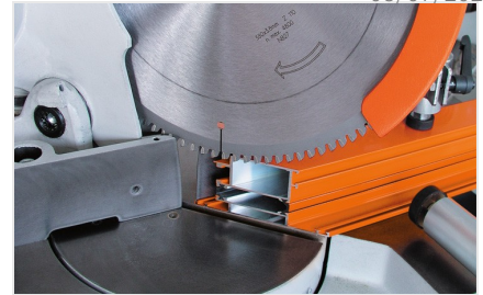
单头斜榫切割机MGS 72/30
