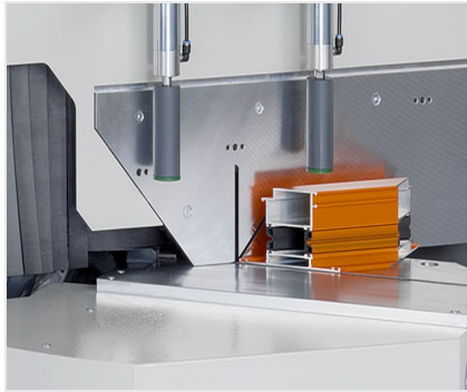
单头斜棒切割机MGS 105
