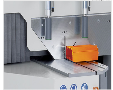
单头斜棒切割机MGS 105
