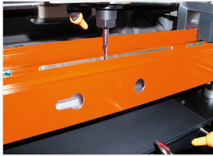
双轴仿形铣床KF 78/23
