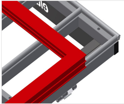
支承面 HT 2000 / HT 2000 E / HT 3000 / HT 3000 E / HT 2045 L / HT 2045 R 带塑料滑条的工作台支承面
