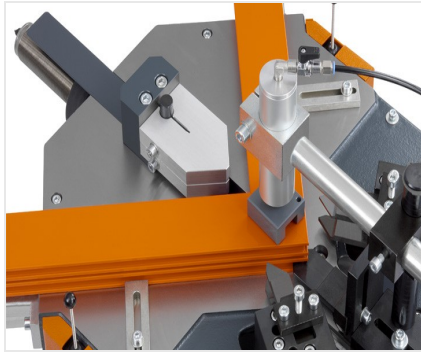
单头组角机EP 120
