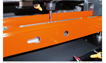
Üç Motorlu Kopya Freze KF 178/10
