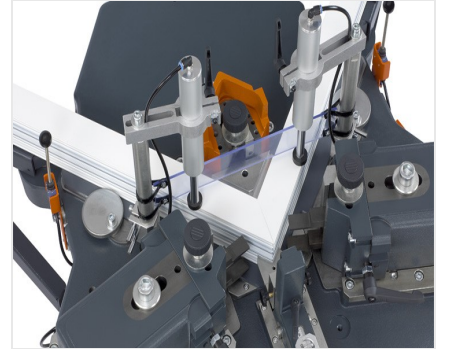
Köşe bağlantı presi EP 124
