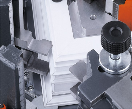
Köşe bağlantı presi EP 124
