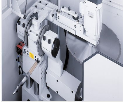
Profil Alıştırma Makinesi AKS 134/00
