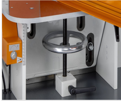
Orta Kayıt Kerme Makinesi AF 223/01
