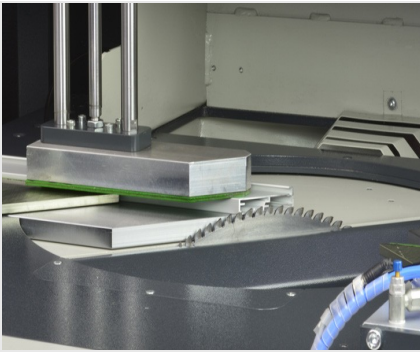
Пильный центр SBZ 616/02
