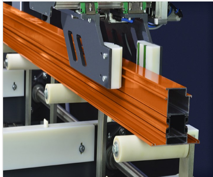
Пильный центр SBZ 616/02
