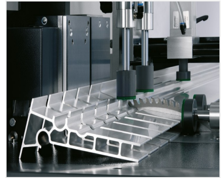
Пильный автомат SAS 142/44
