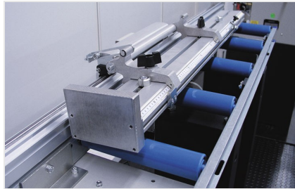
Упорно-измерительная система MMS 200
