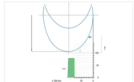
Máquina de corte em V KS 101/30
