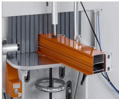
Fresa de malhetar AF 223/01
