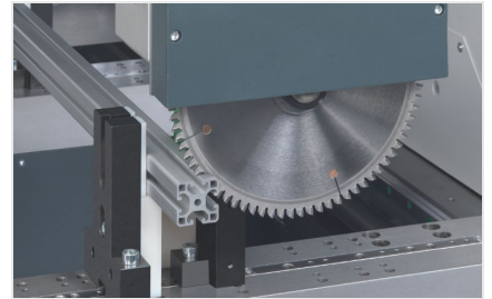
SBZ 140 Profilbewerkingscentrum
