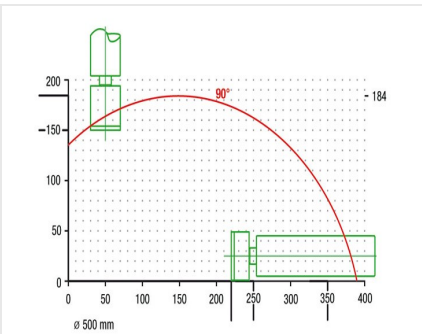
Zaagautomaat SAS 142/44
