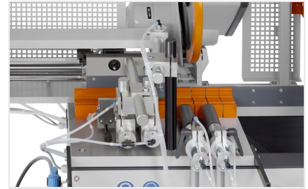
Zaagautomaat SA 73/36
