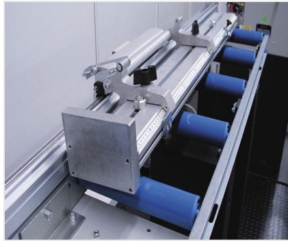
Aanslag- en meetsysteem MMS 200
