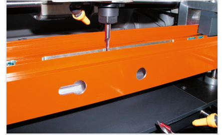
Driespindel- kopieerfreemachine KF 178/10
