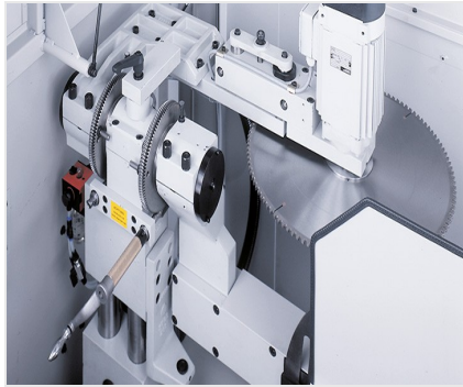
Uithoekzaagmachine AKS 134/00
