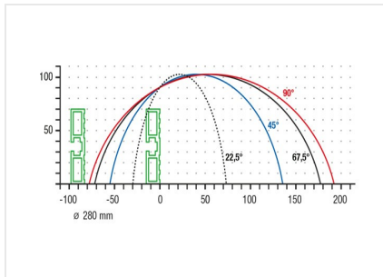
台式锯床TS 161/21 切割图TS 161/21
