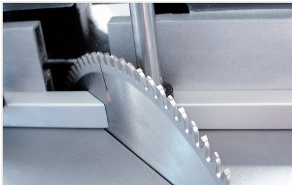
台式锯床TS 161/21
