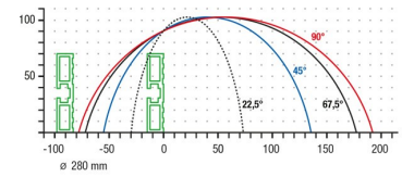
台式锯床TS 161
