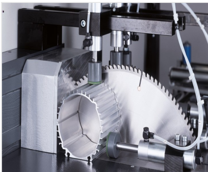
自动锯切机SA 142/37
