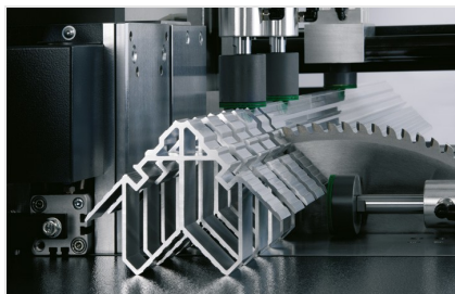
自动锯切机SA 142/38
