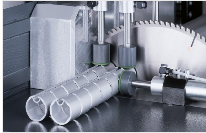
自动锯切机SA 142/37
