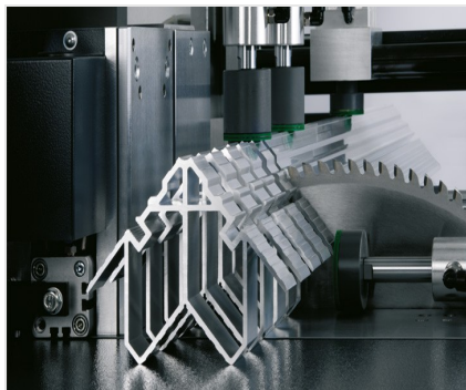
自动锯切机SA 142/38
