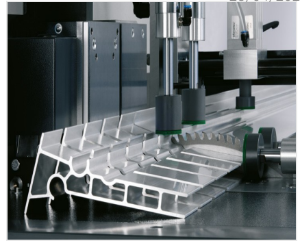
自动锯切机SA 142/38
