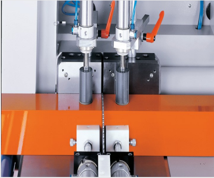
单头斜榫切割机MGS 142/31 切割缝开口
