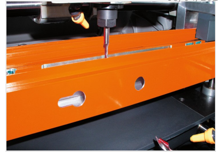
双轴仿形铣床KF 78/23
