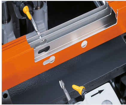
双轴仿形铣床KF 78/23
