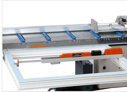
玻璃压条切割机GLS 192/07
