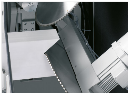
端面角切割机AKS 134/64
