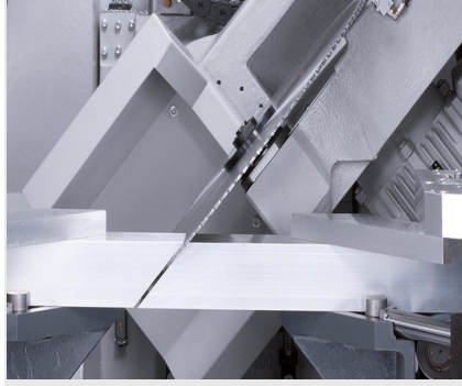
Profil İşleme Merkezi SBZ 631
