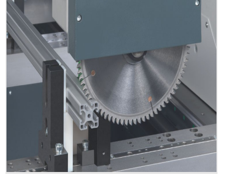
SBZ 140 Profil İşleme Merkezi
