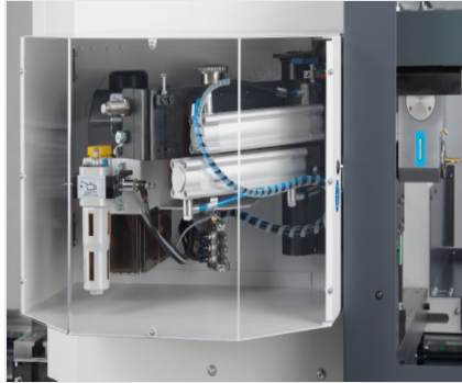
SBZ 140 Profil İşleme Merkezi
