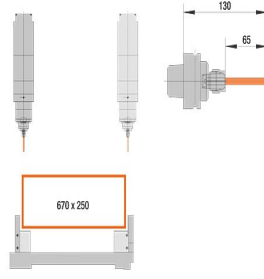
SBZ 140 Profil İşleme Merkezi
