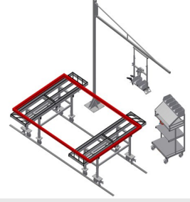
Çift Montaj İstasyonları MSA 2400 + G 3000 + S 3000 + WKW 800
