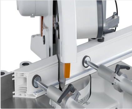
Tek Başlı Testere MGS 73/33
