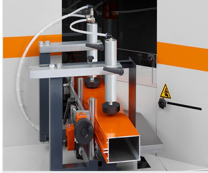
Profil Alıştırma Makinesi AKS V-550
