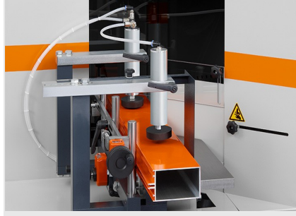
Profil Alıştırma Makinesi AKS V-550
