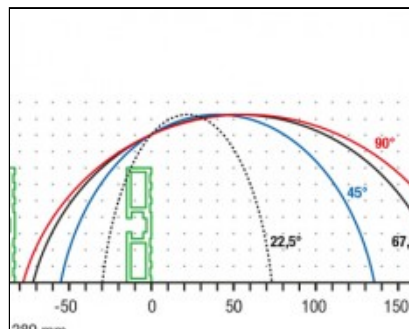
Настольная пила TS 161
