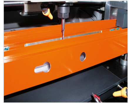
Двухшпindelный копировально- фрезерный станок KF 78/23
