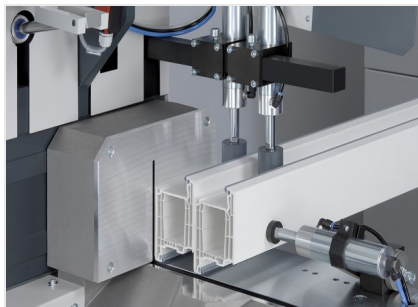
06. Двойная усорезная пила DG 142 XL
