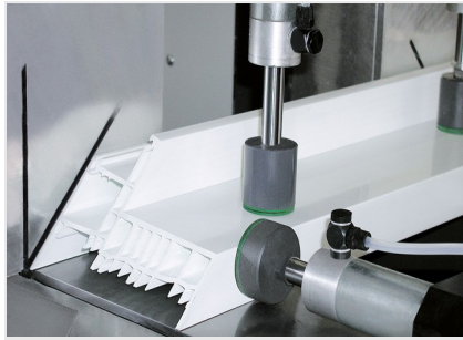
03. Двойная усорезная пила DG 142 XL
