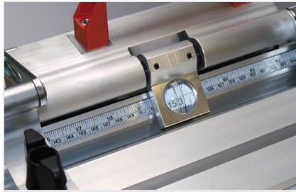
Упорно-измерительная система AMS 200
