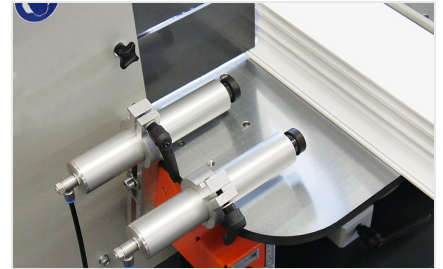
Фрезерный станок для фрезерования торцов AF 222/02
