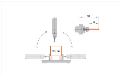
Centro estático SBZ 140 eluCam
