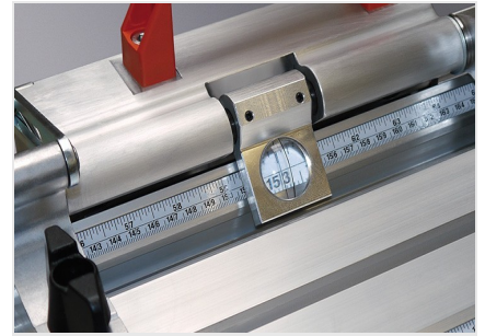
Sistema de batente e medição MMS 200
