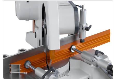
Máquina de corte angular MGS 73/33
