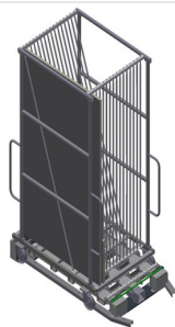
Carro de divisões para vidro GFW 15 + Estação de elevação de vidro GHS 15
