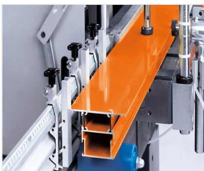
Fresa-copiadora de 1 cabeça AS 170/10
