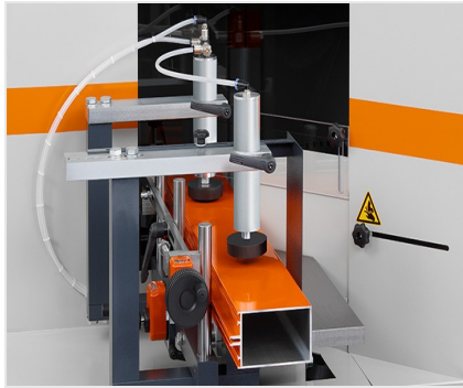
Máquina de corte e malhete AKS V-550
