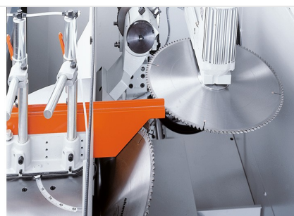
Máquina de corte e malhete AKS 134/00
