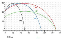
Piła obrotowa MGS 105
