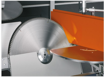
Piły do wycięć klinowych AKS 134/64
