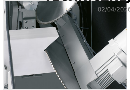
Piły do wycięć klinowych AKS 134/64
