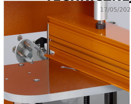
Frezarka do słupków AF 223/01
